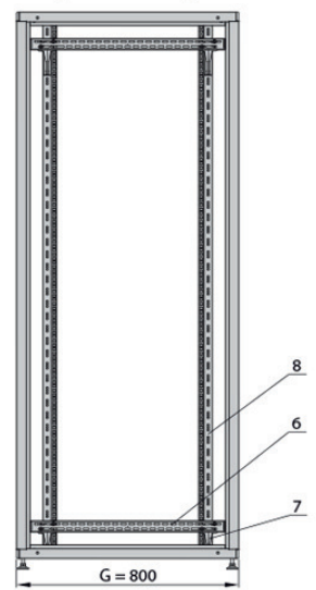
Seitenansicht (Schrantiefe 800 mm)
