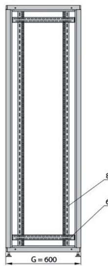
Seitenansicht (Schrantiefe 600 mm)
