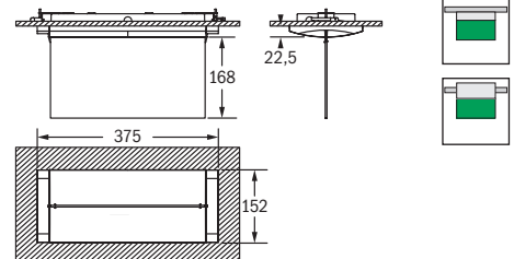
Decken-Ausnehmung 370 x 130
