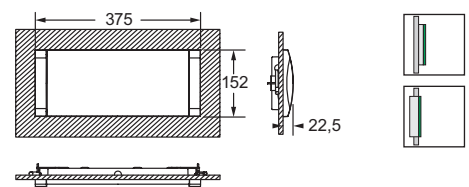
Wand-Ausnehmung 370 x 130
