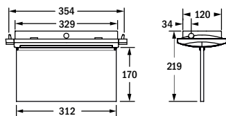
Deckenanbau
