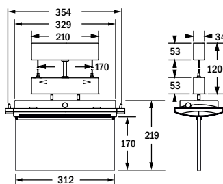
Deckenanbau
