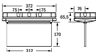
Deckeneinbau Massivdecken
