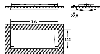
Wandeinbau Hohlwände
