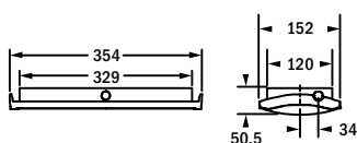
Wandanbau
