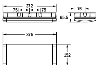
Deckeneinbau Massivdecken
