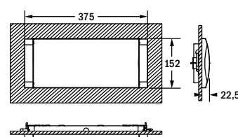
Wandeinbau Hohlwände
