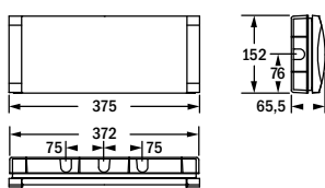
Wandeinbau Massivwände
