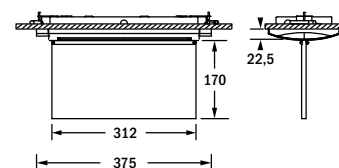
Deckeneinbau Hohldecken
