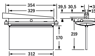
Deckeneinbau Massivdecken
